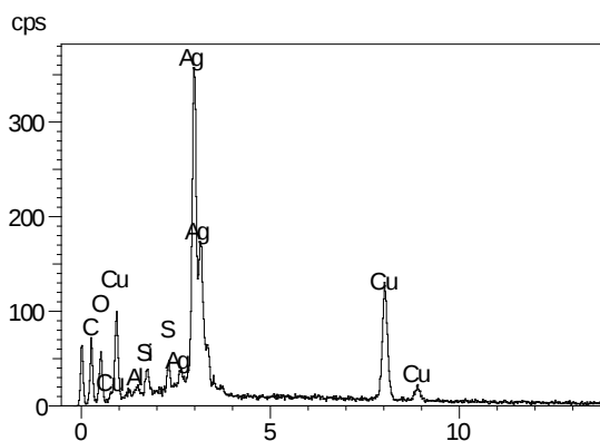
Tav. XV Analisi su un particolare della superficie dove, con elettroni retrodiffusi, si evidenzia la presenza di zone ossidate (scure nell'immagine di sinistra), con formazione di solfuro di argento: sulla destra lo spettro EDS, relativo al punto evidenziato dalla croce, mostra la presenza di zolfo (S), oltre a rame (Cu), argento (Ag) e tracce organiche (C, O).
