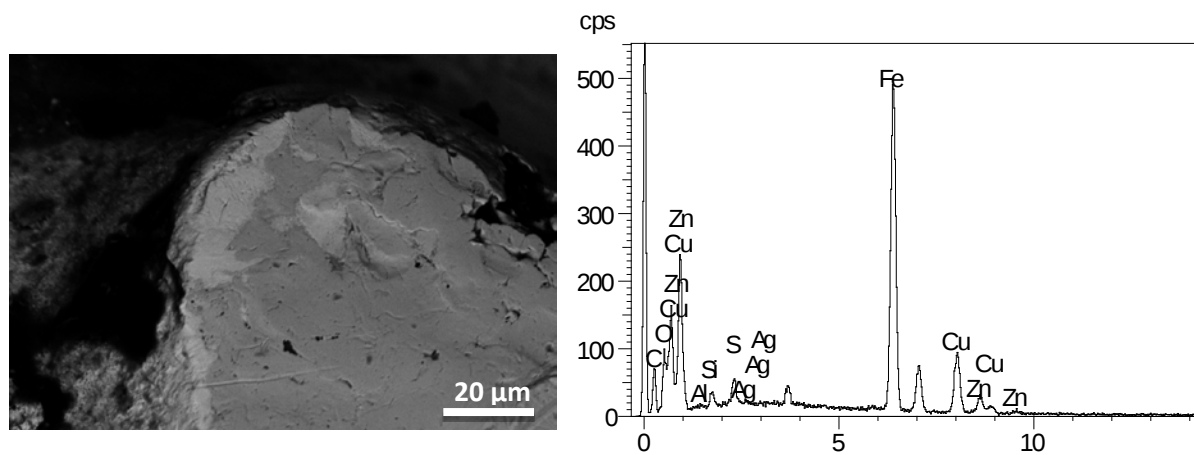
Tav. XVIII Dalla microfotografia (immagine sulla sinistra, elettroni retrodiffusi) si può osservare l'usura superficiale della vite e il permanere in alcune zone (aree più chiare nell'immagine) di resti della finitura in ottone.
