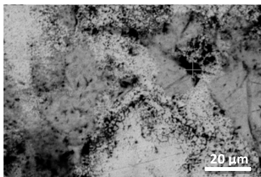
Tav. XV Analisi su un particolare della superficie dove, con elettroni retrodiffusi, si evidenzia la presenza di zone ossidate (scure nell'immagine di sinistra), con formazione di solfuro di argento: sulla destra lo spettro EDS, relativo al punto evidenziato dalla croce, mostra la presenza di zolfo (S), oltre a rame (Cu), argento (Ag) e tracce organiche (C, O).
