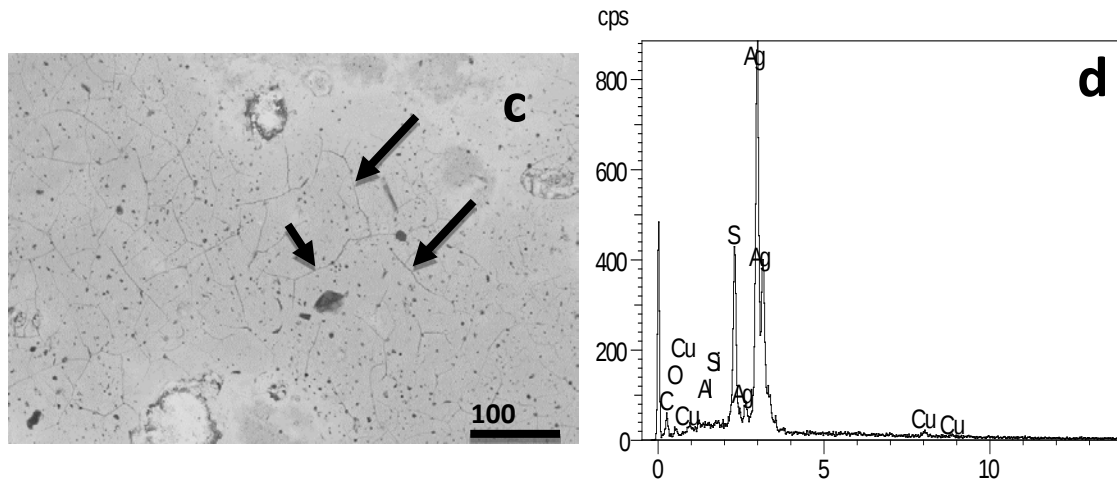
Tav. XVII Immagini a diversi ingrandimenti in elettroni retrodiffusi (XVII c) della zona scura del sigillo, e relativo spettro EDS (XVII d). Sono evidenti i bordi grano, evidenziati dalle frecce, che testimoniano per un probabile degrado da intervento.
