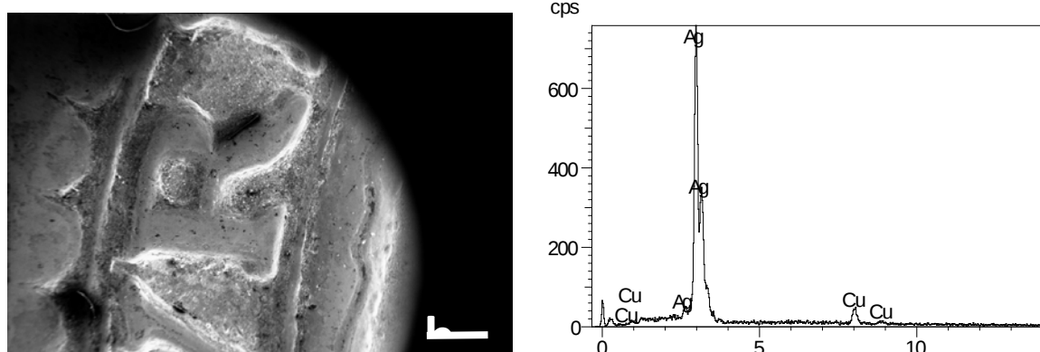
Tav. XVI Particolare del sigillo (a sinistra, elettroni secondari) con relativa analisi EDS media sull'area (a destra).
