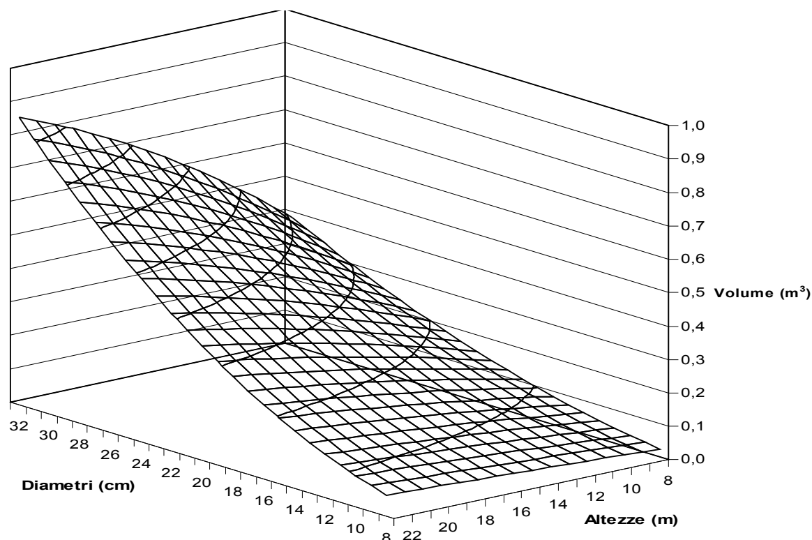
Fig. 2 - Andamento del volume al variare del diametro e dell'altezza.
